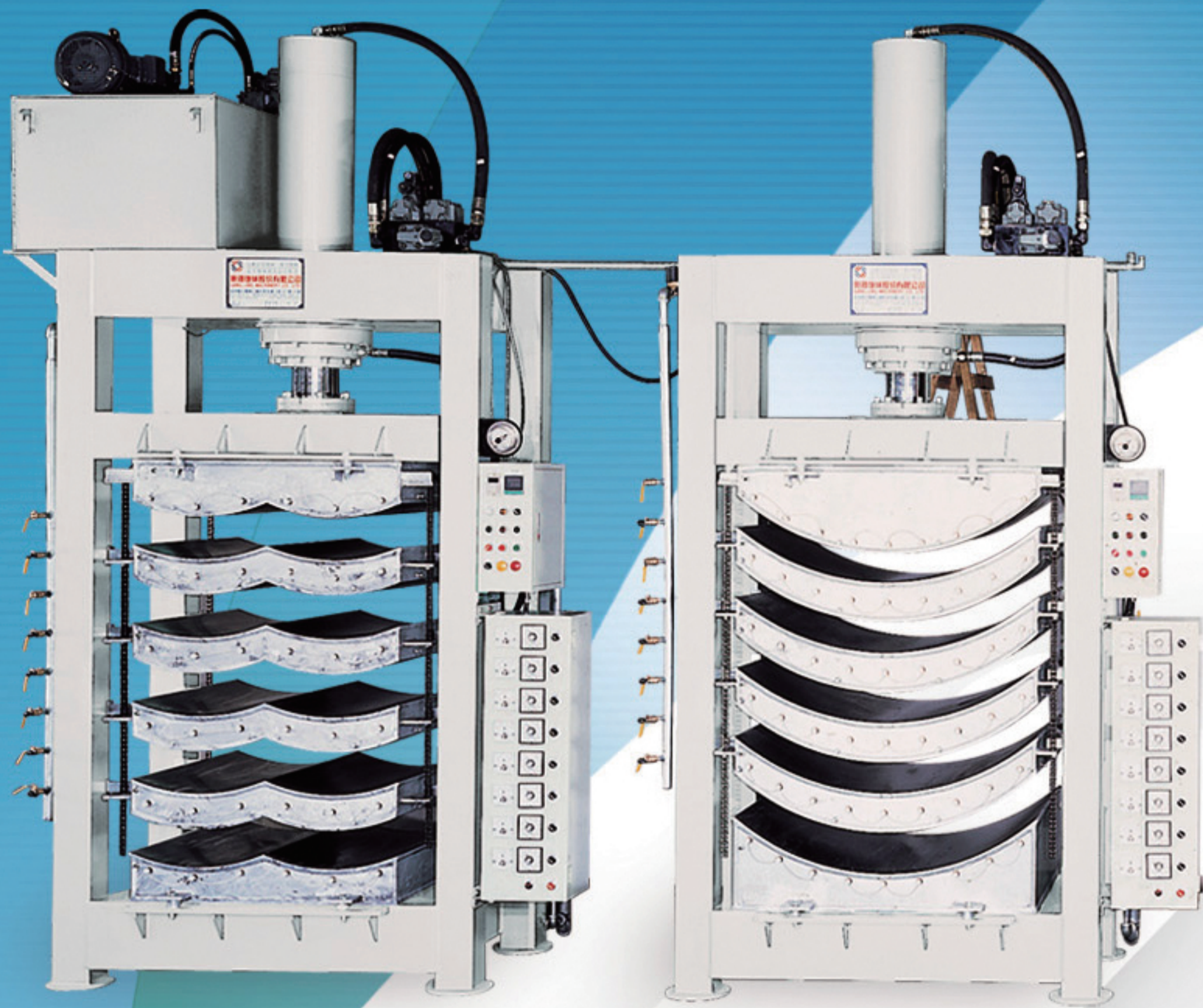
油壓曲木成型機 Hydraulic Bentwood Forming Machine
